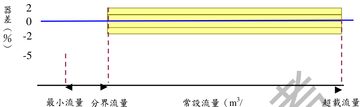
【圖 3：速度型橫軸奧多曼式水量計性能曲線圖】
